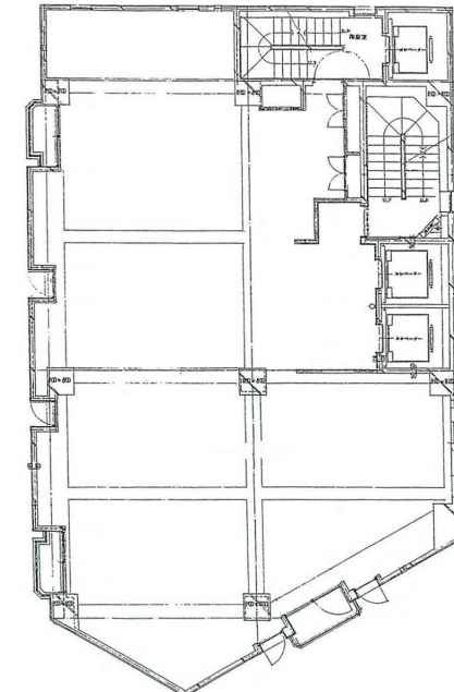
3~6階平面図
