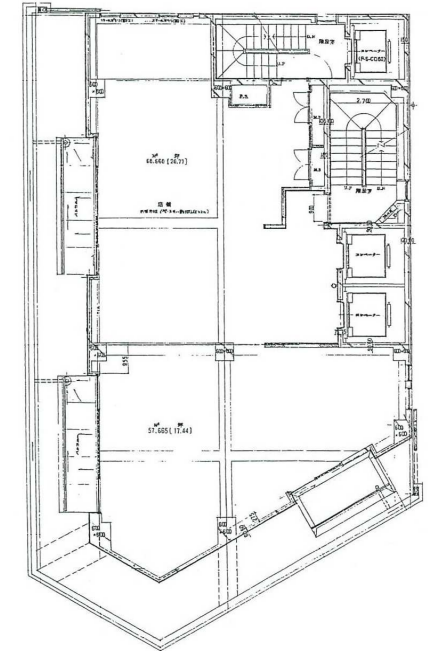
8階平面図
